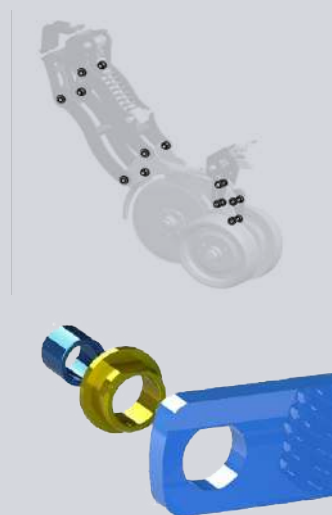
Sistema de bucha e contra-bucha nas articulações
