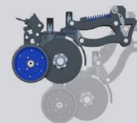
Disco duplo defasado de ângulo fechado
